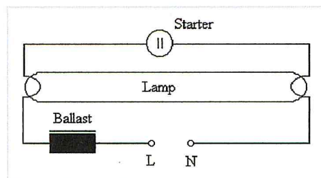
Схема включения
